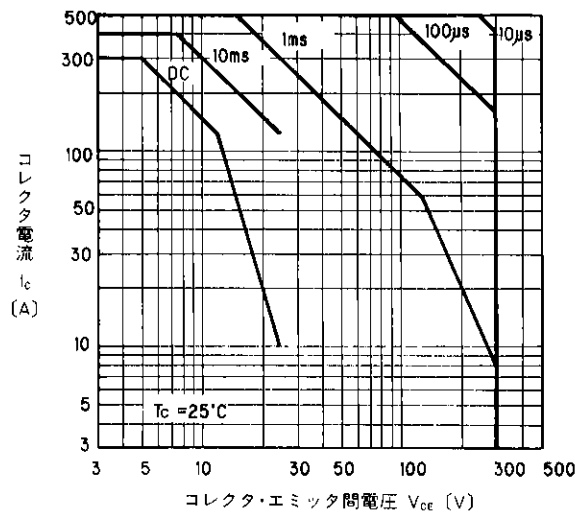
安全動作領域特性
