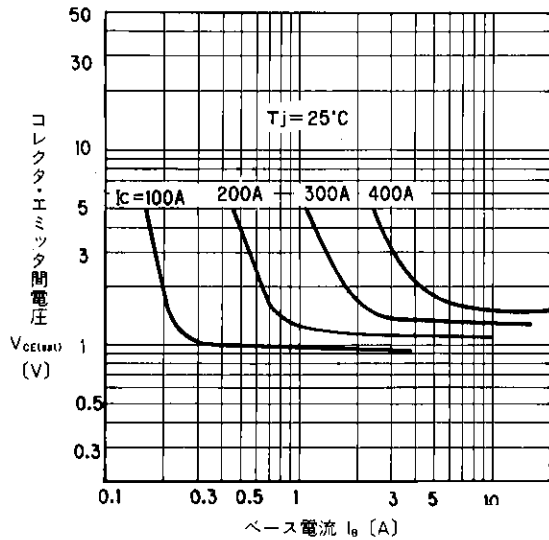
出力特性
