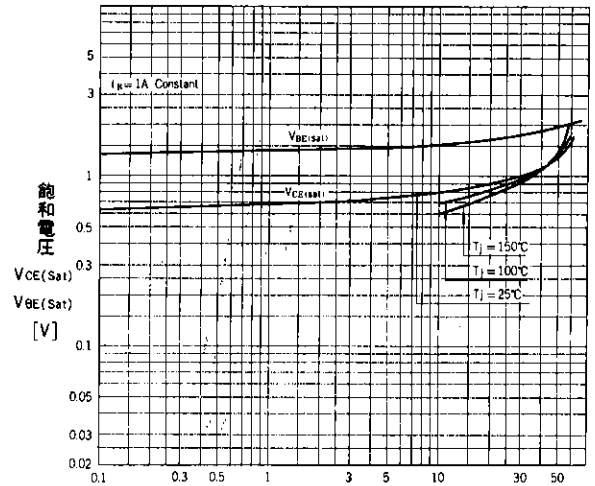
コレクタ電流 I_c [A] 飽和電圧—コレクタ電流特性 Base and Collector Saturation Voltage
